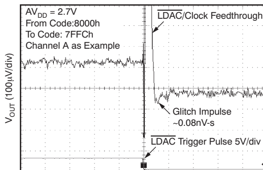
GLITCH ENERGY: 2.7V, 4LSB STEP, FALLING EDGE
