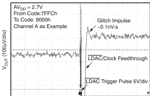
GLITCH ENERGY: 2.7V, 4LSB STEP, RISING EDGE
